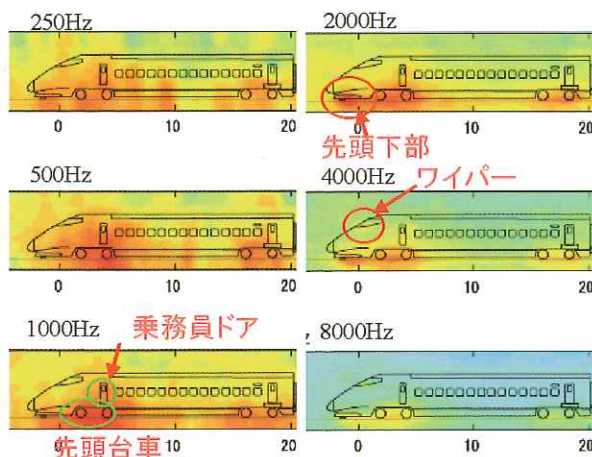
音源分布測定結果例
