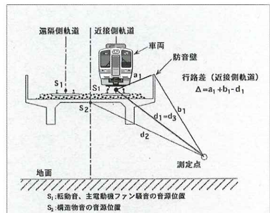
在来鉄道騒音の音源と伝搬経路
