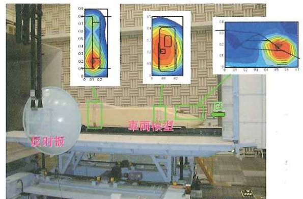
空力騒音に関する風洞試験例
