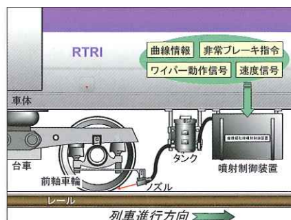
車輪/レール摩擦緩和システム「FRIMOS」
