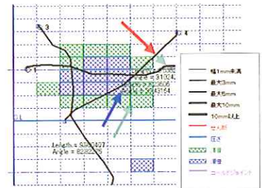
トンネル健全度診断システム
