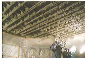
吹付け修復工法 「JOT'S Crete (ジョッツ クリート)」
