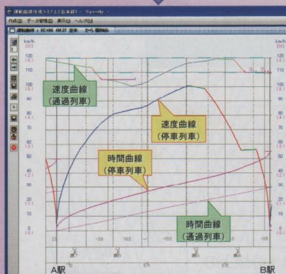
運転曲線図作成結果
